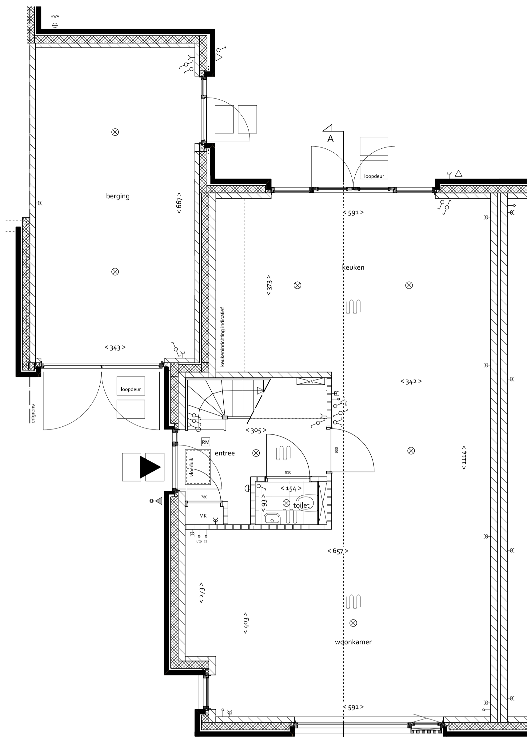
BEGANE GROND 1:50
