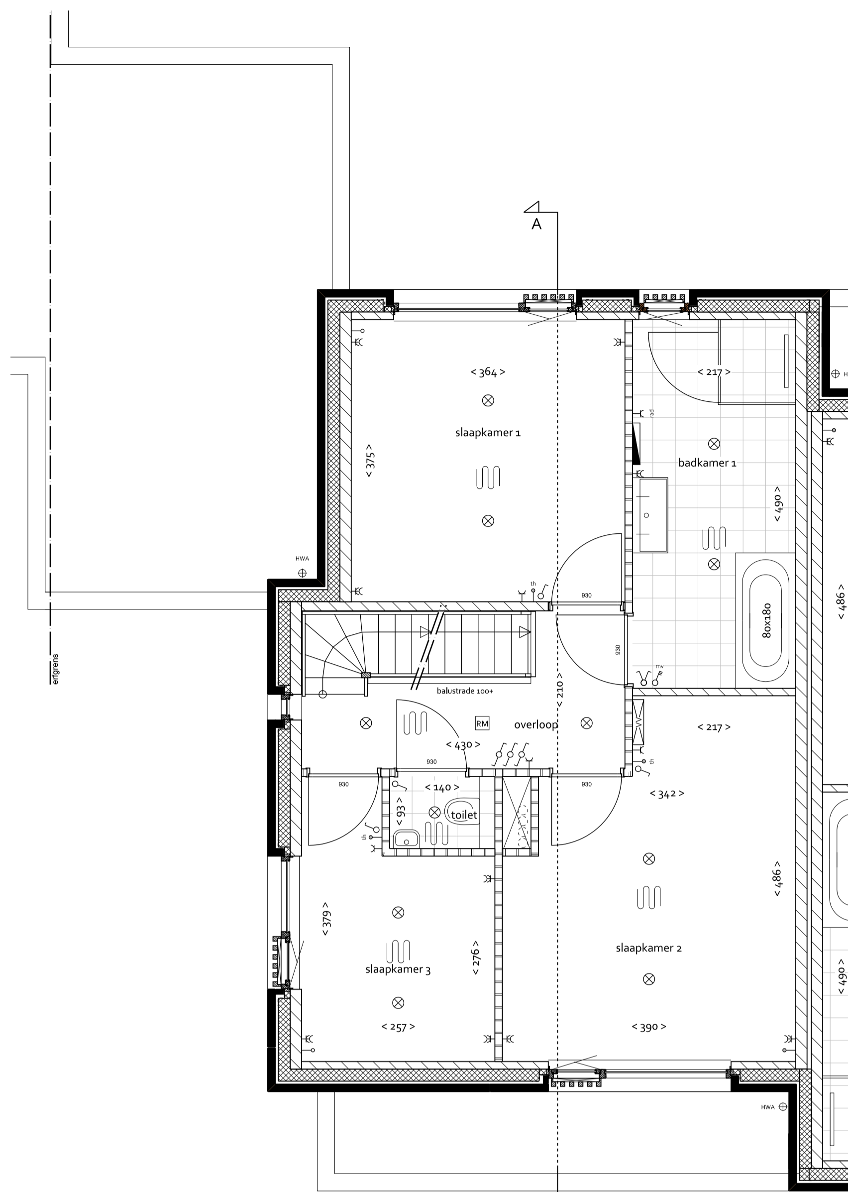
EERSTE VERDIEPING 1:50
