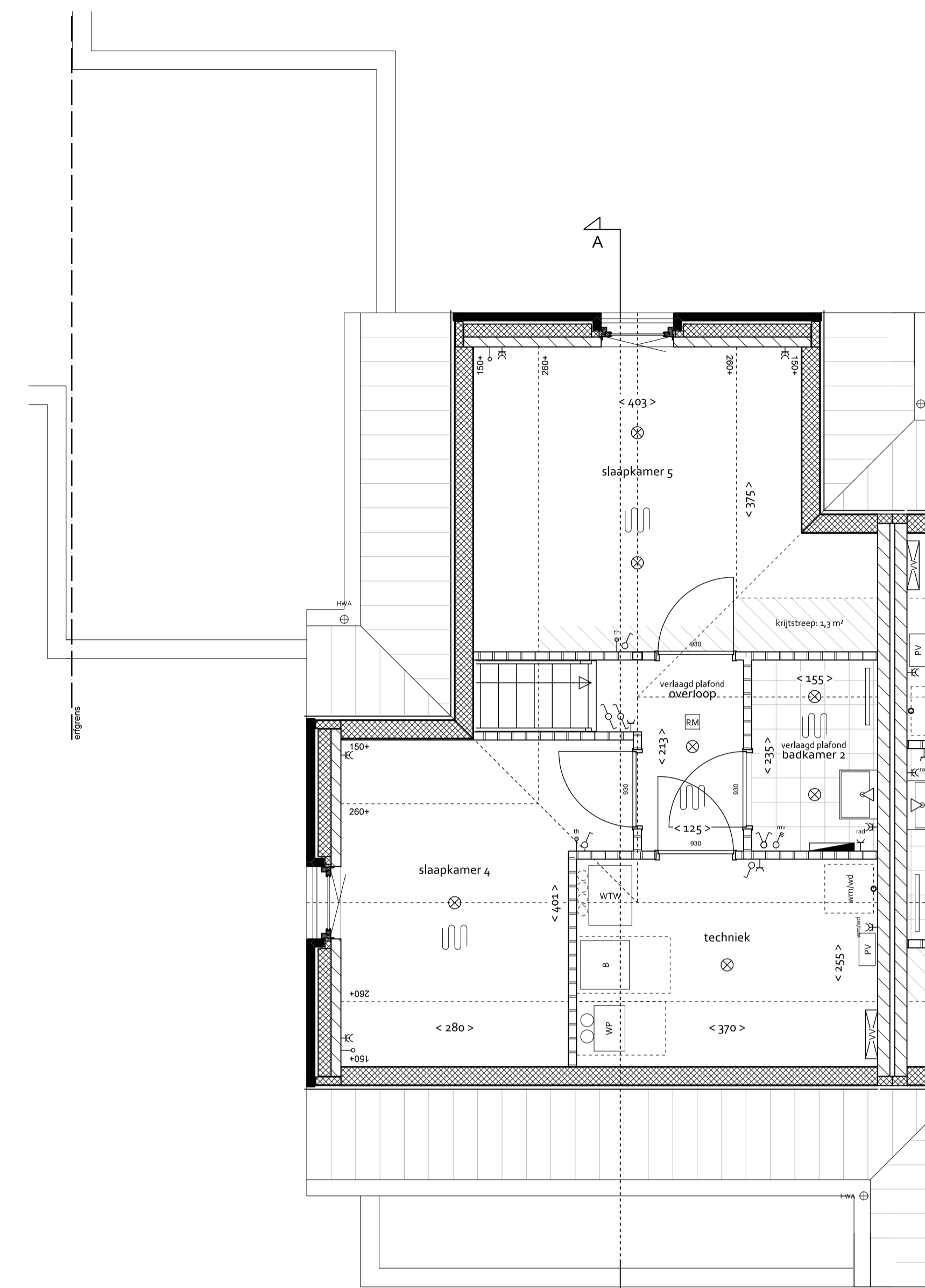
TWEDE VERDIEPING 1:50
