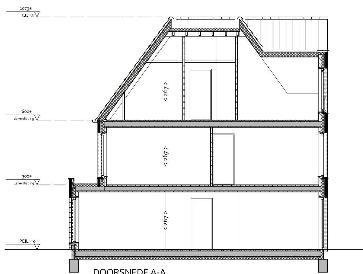
DOORSNEDEN A-A 1:100
