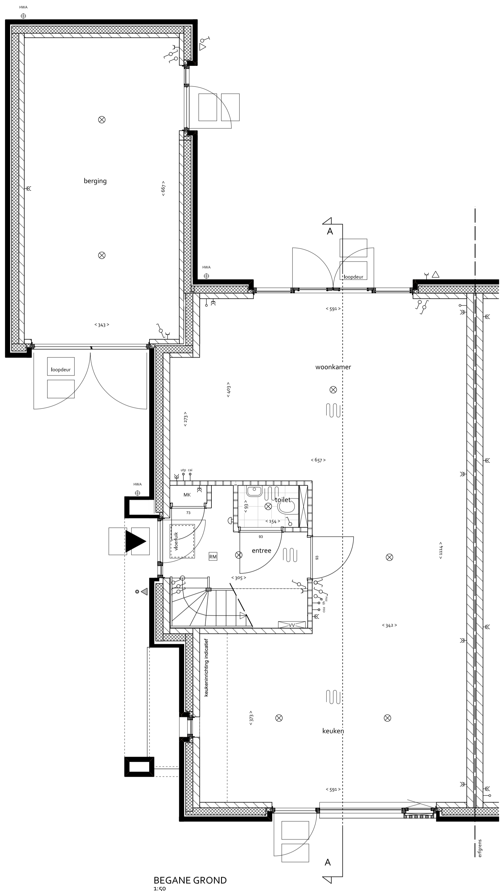
BEGANE GROND 1:50
