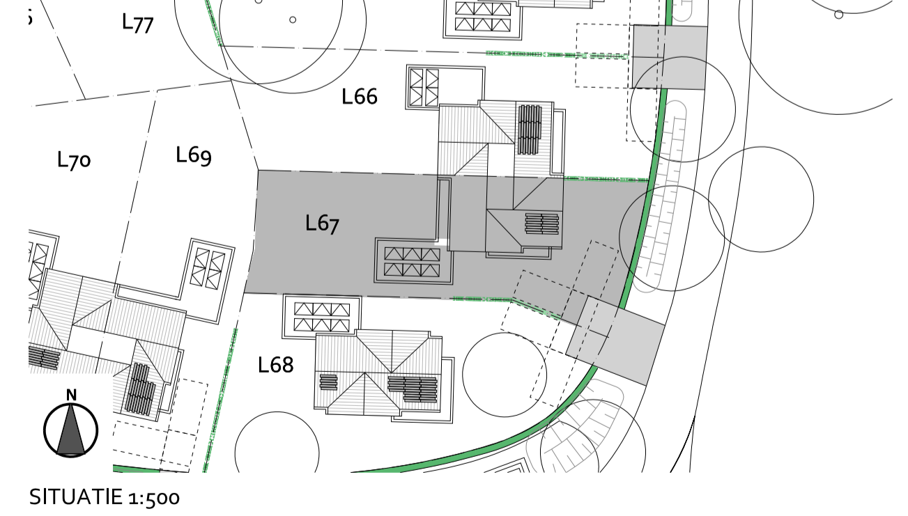
SITUATIE 1:500
