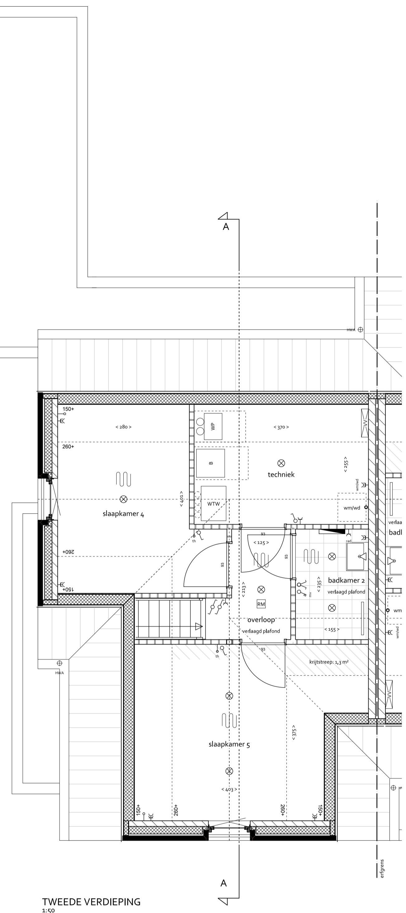
TWEEDE VERDIEPING 1:50
