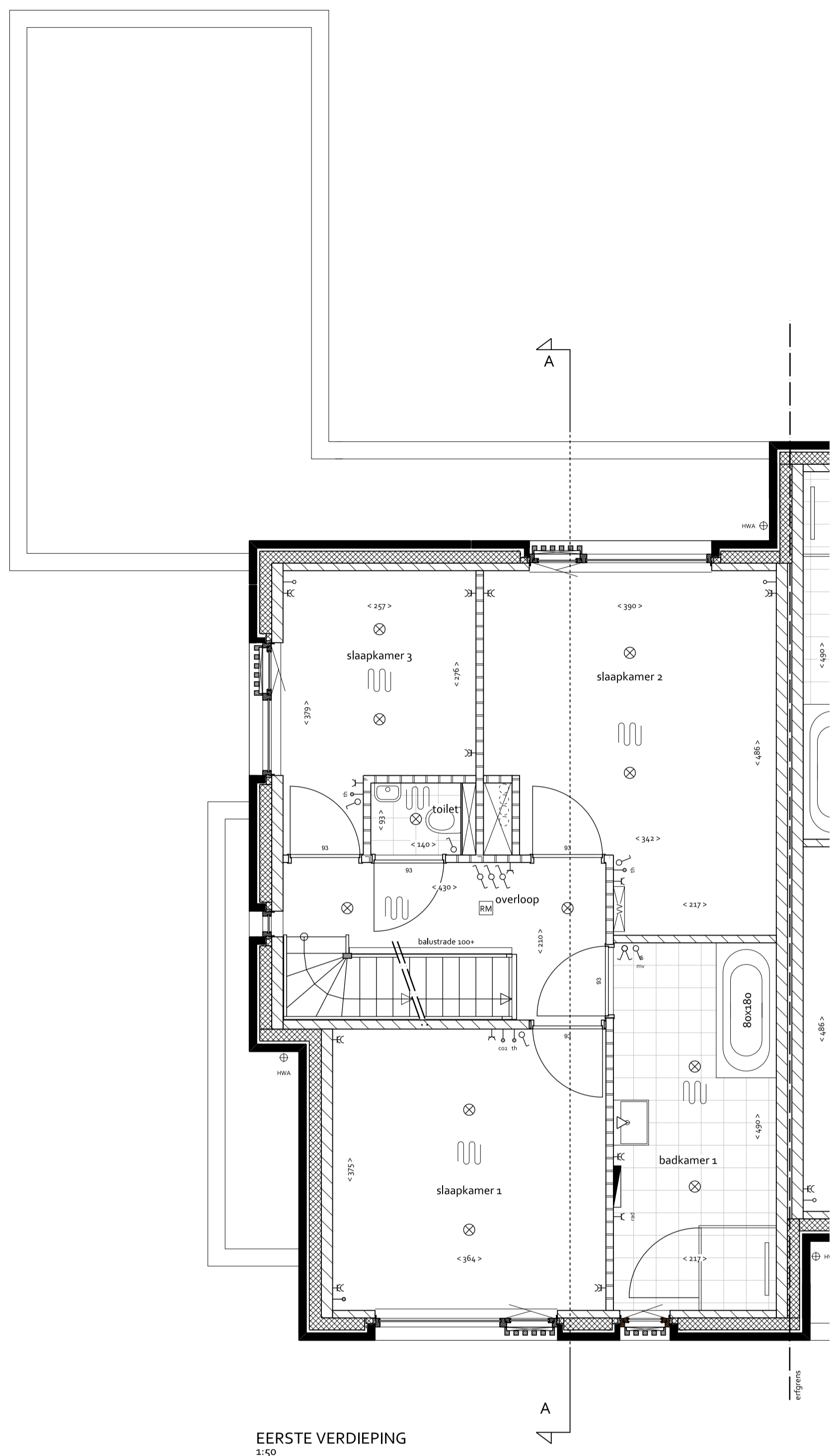
EERSTE VERDIEPING 1:50
