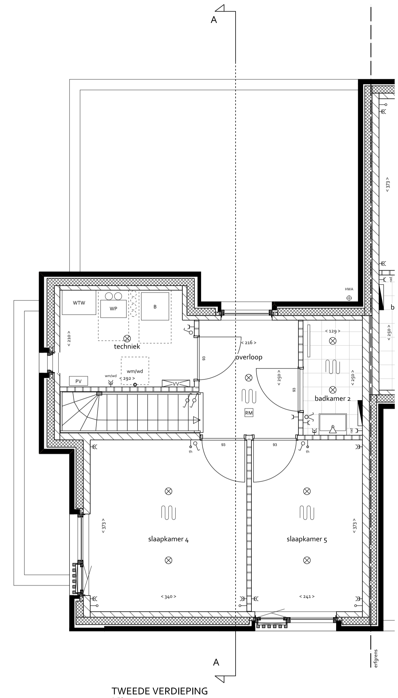
TWEDE VERDIEPING 1:50
