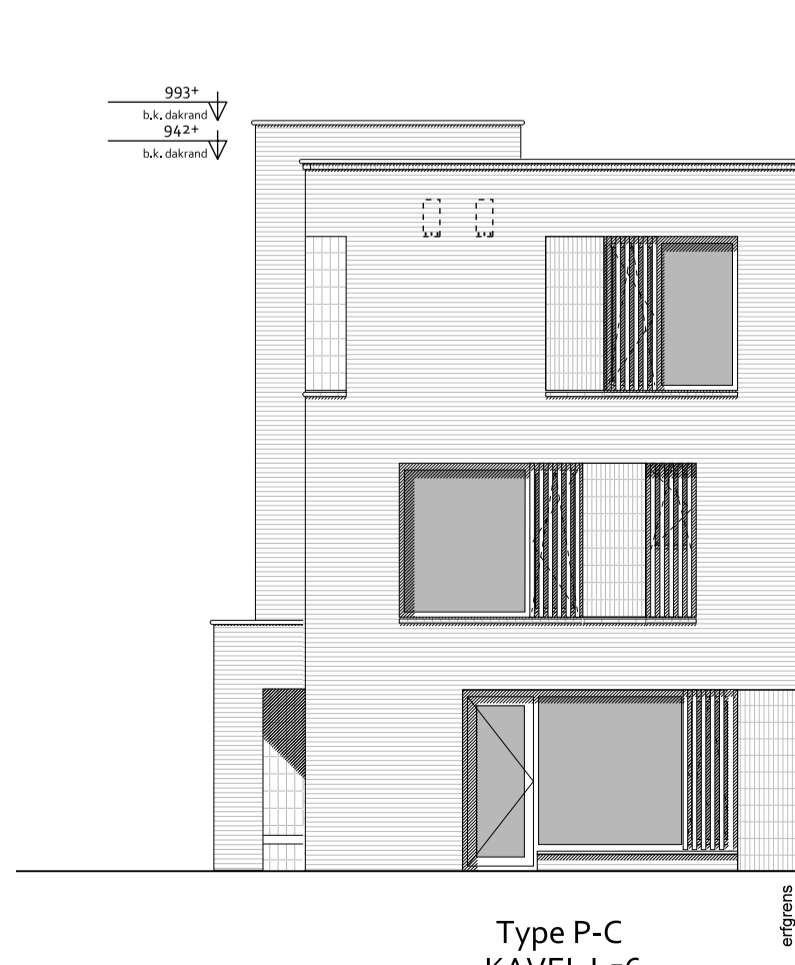
VOORGEVEL 1:100
