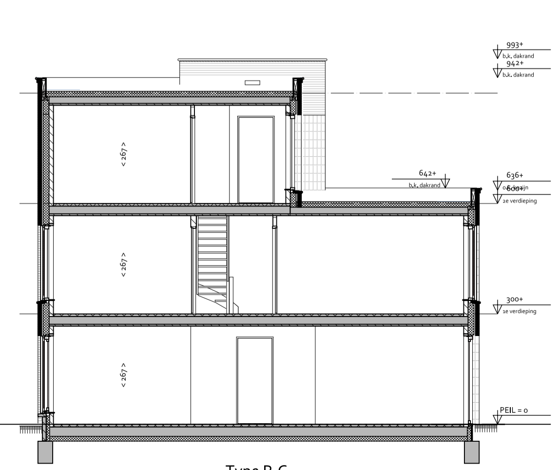
DOORSNEDE A-A 1:100
