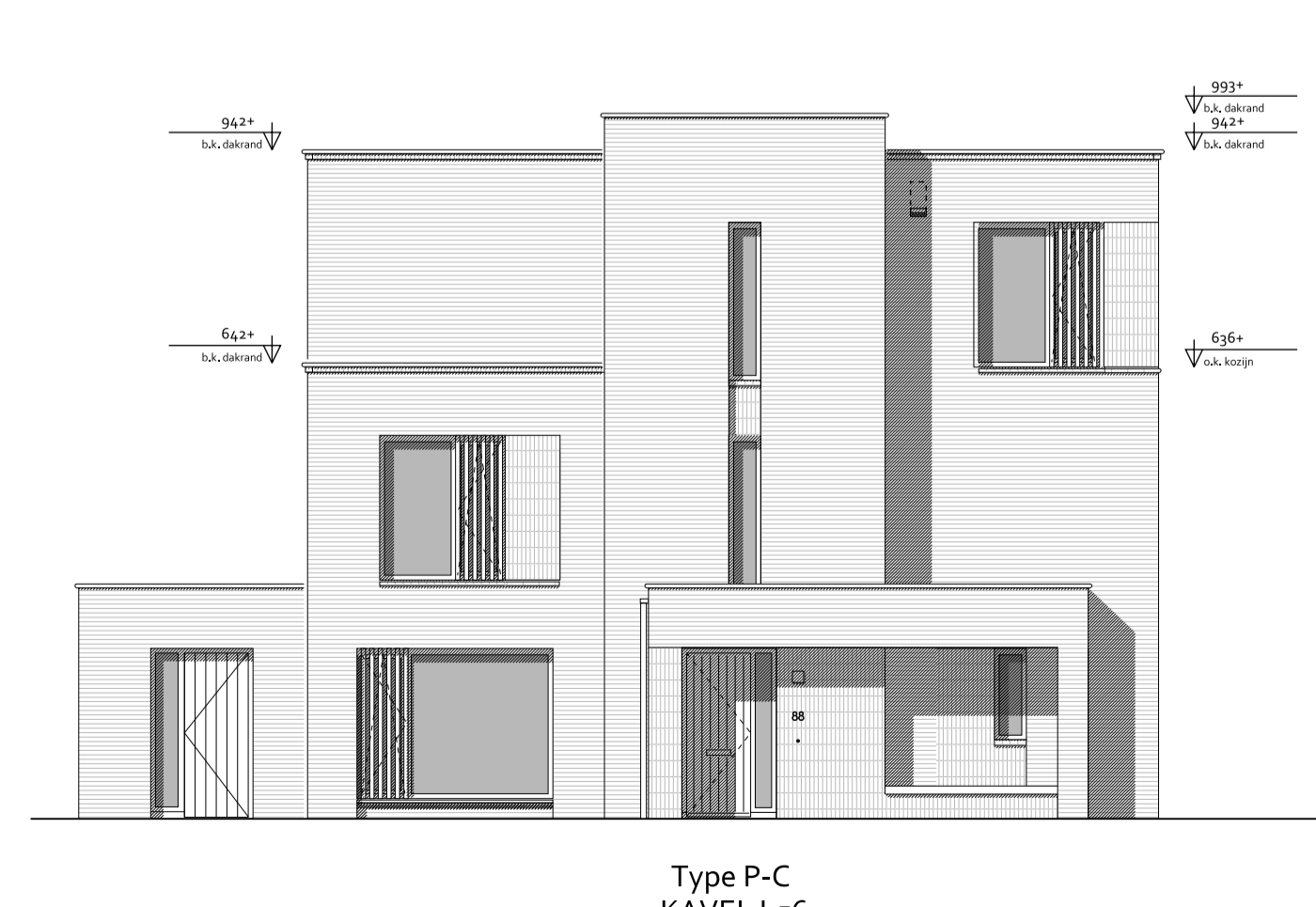
LINKER ZIJGEVEL 1:100
