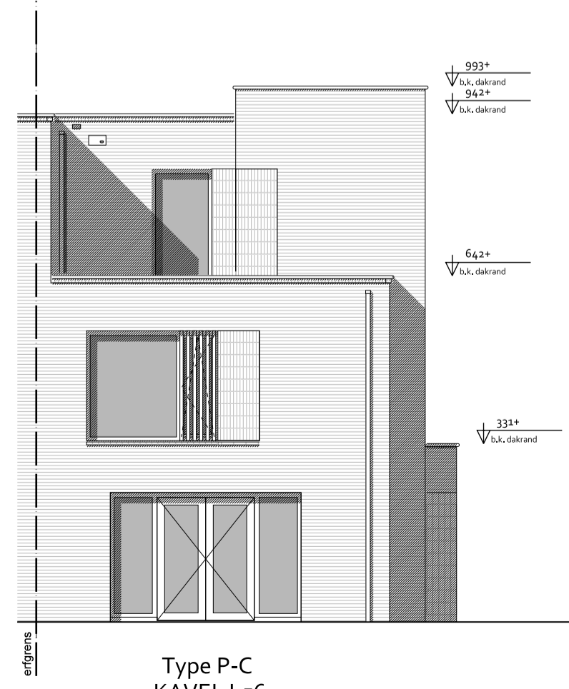
ACHTERGEVEL 1:100
