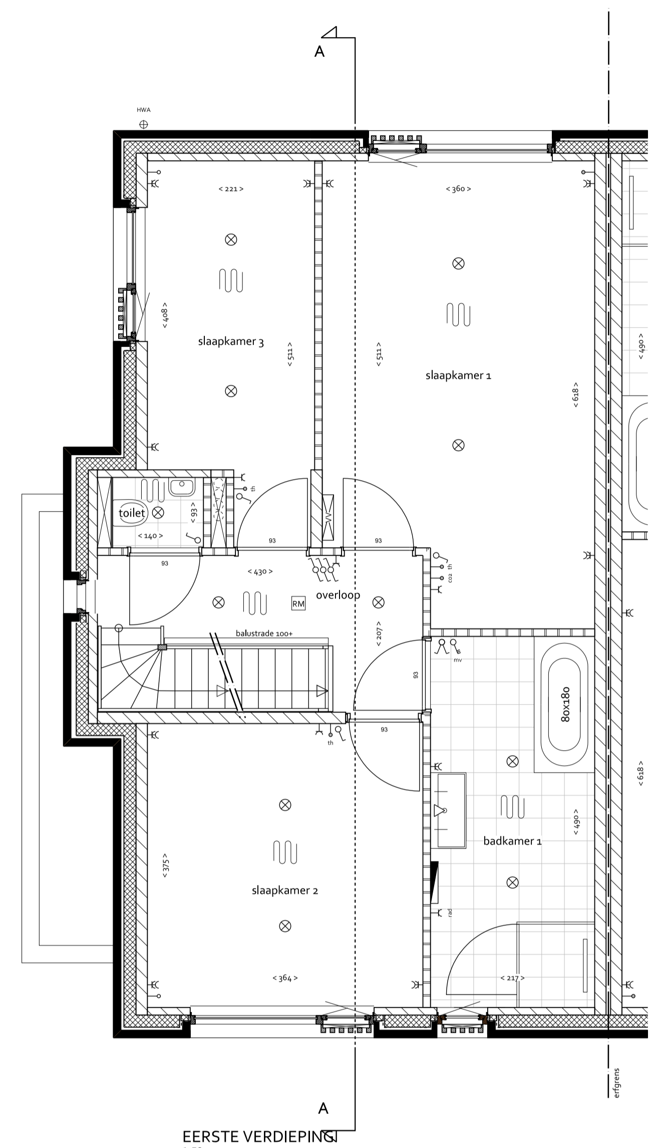
EERSTE VERDIEPING 1:50
