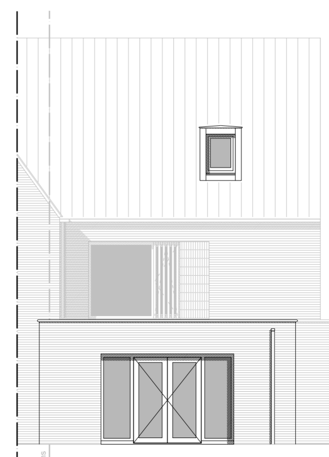
aanzicht uitbouw en dakkapel
