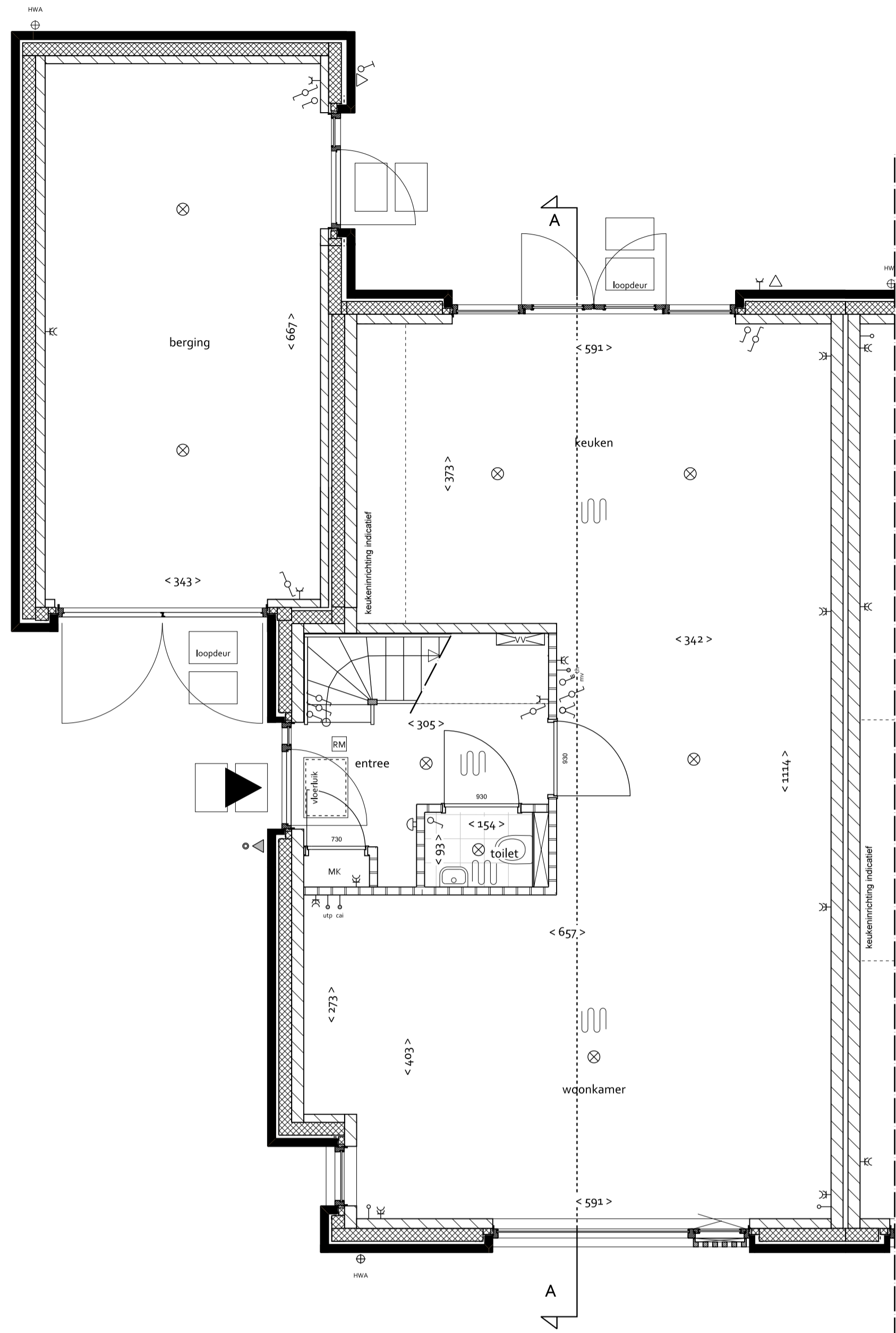
BEGANE GROND 1:50
