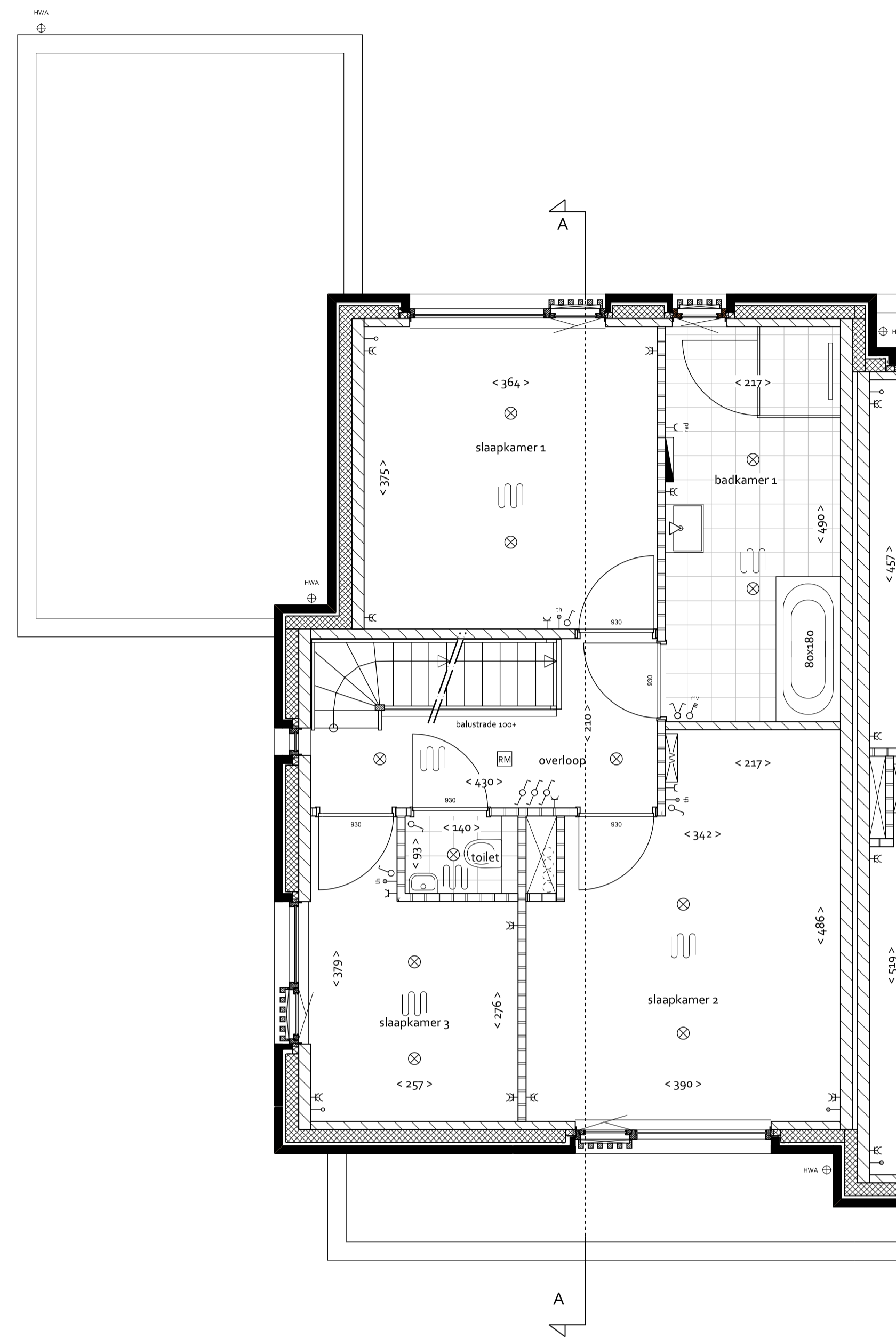
EERSTE VERDIEPING 1:50
