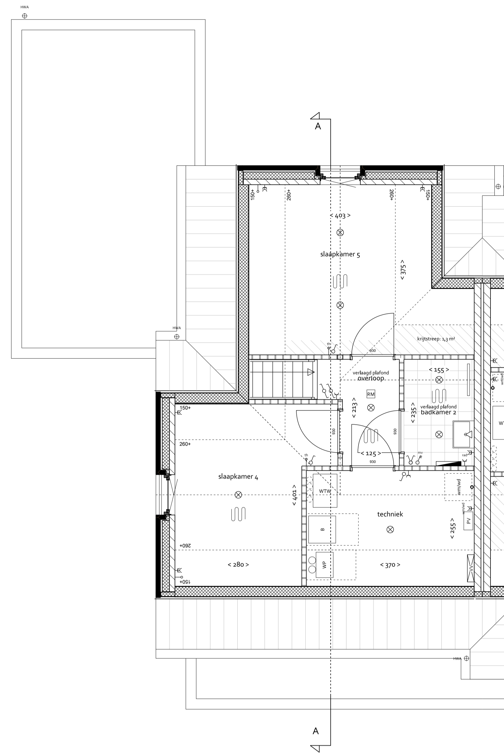
TWEDE VERDIEPING 1:50
