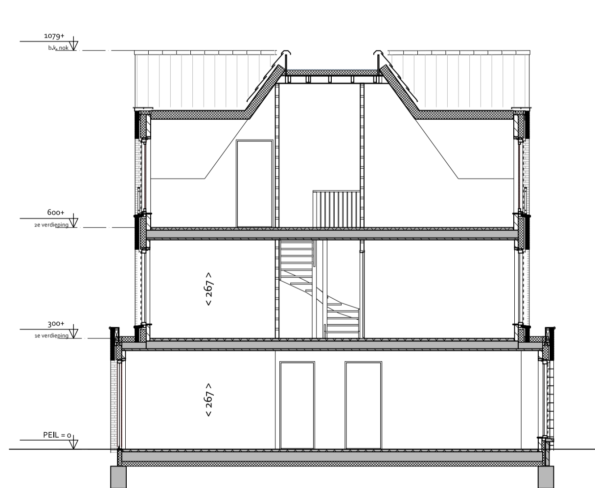
DOORSNEDE A-A 1:100
