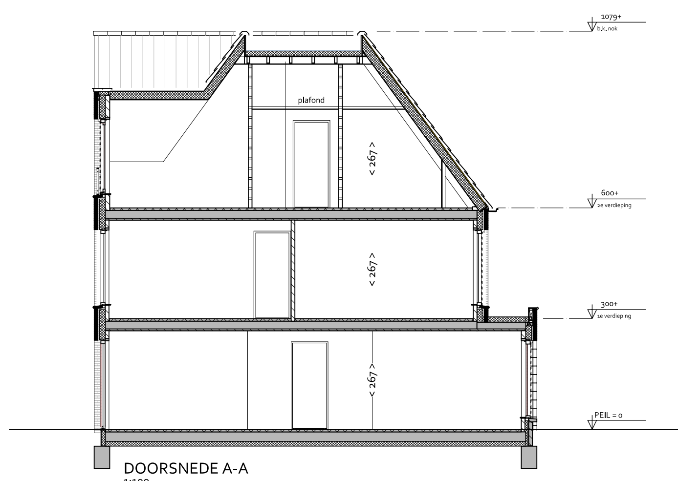
DOORSNEDE A-A 1:100
