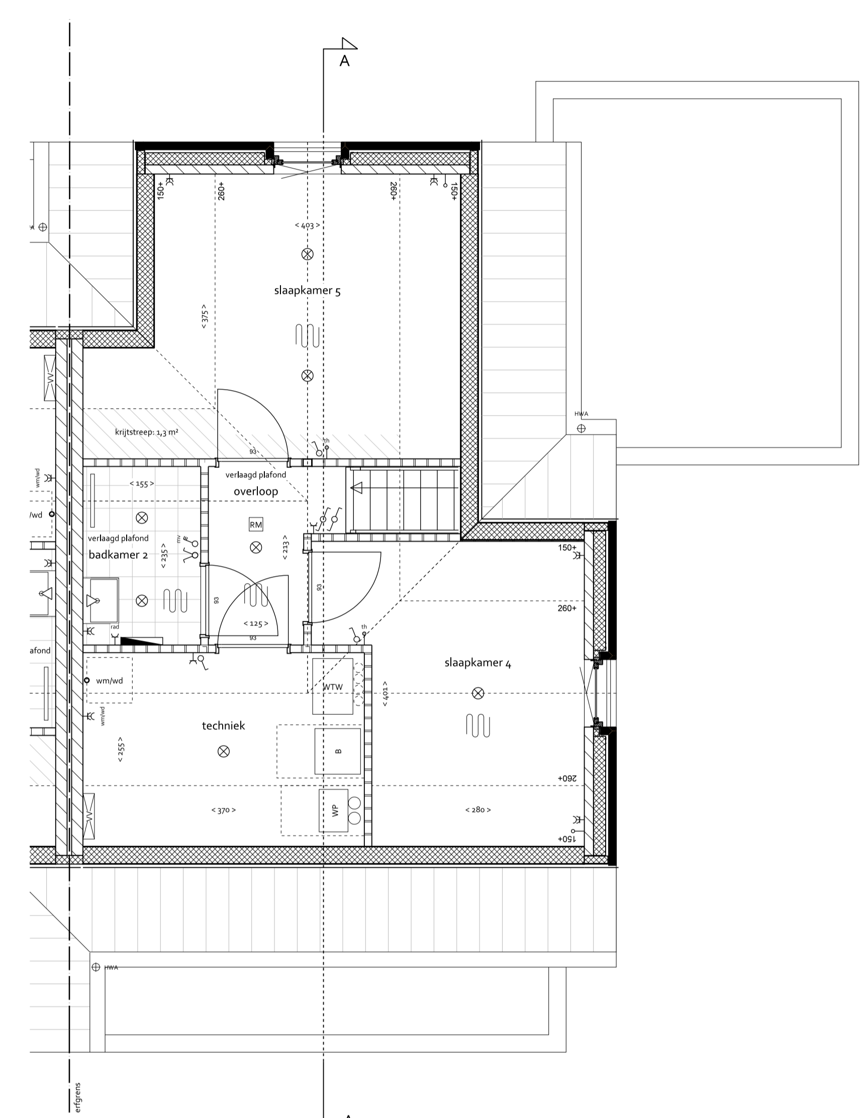
TWEEDE VERDIEPING 1:50
