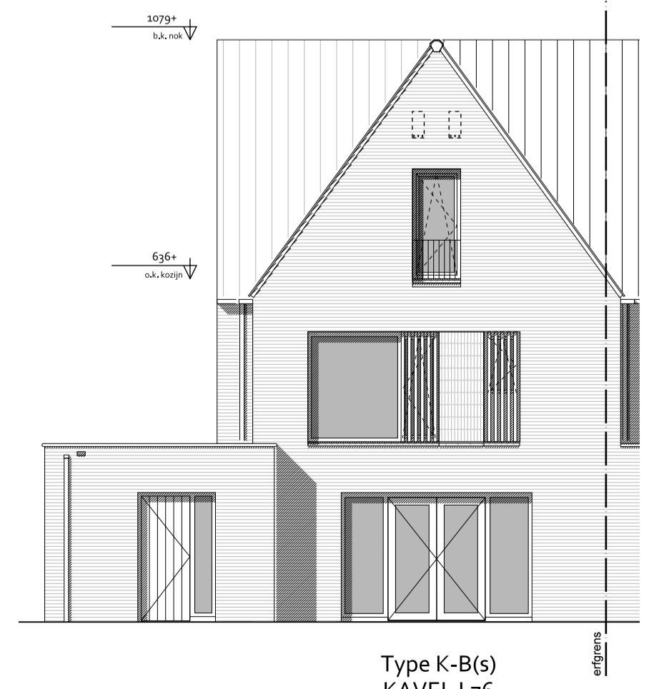
Type K-B(s) KAVEL L76 ACHTERGEVEL 1:100
