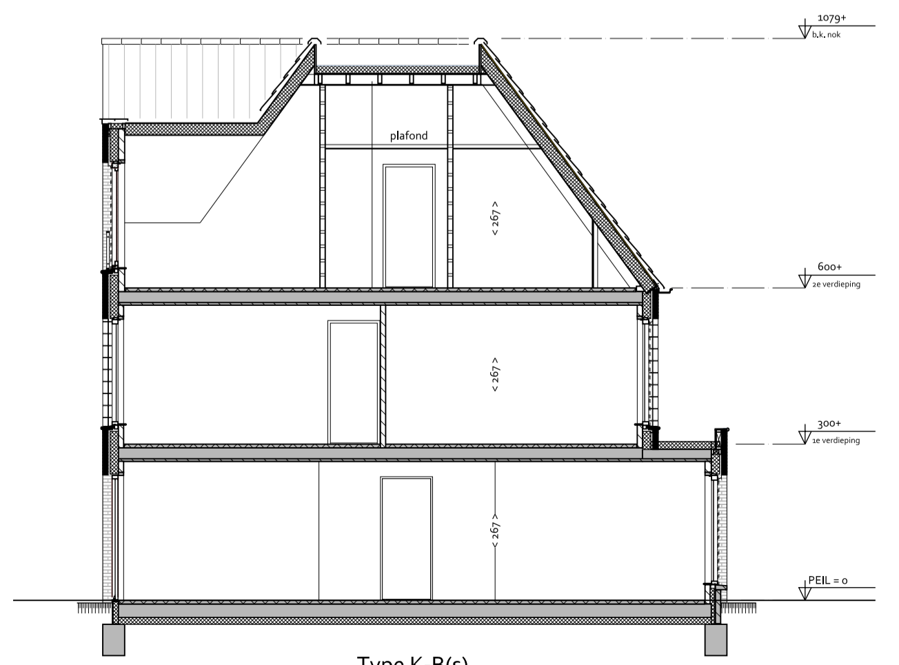
Type K-B(s) DOORSNED E A-A 1:100
