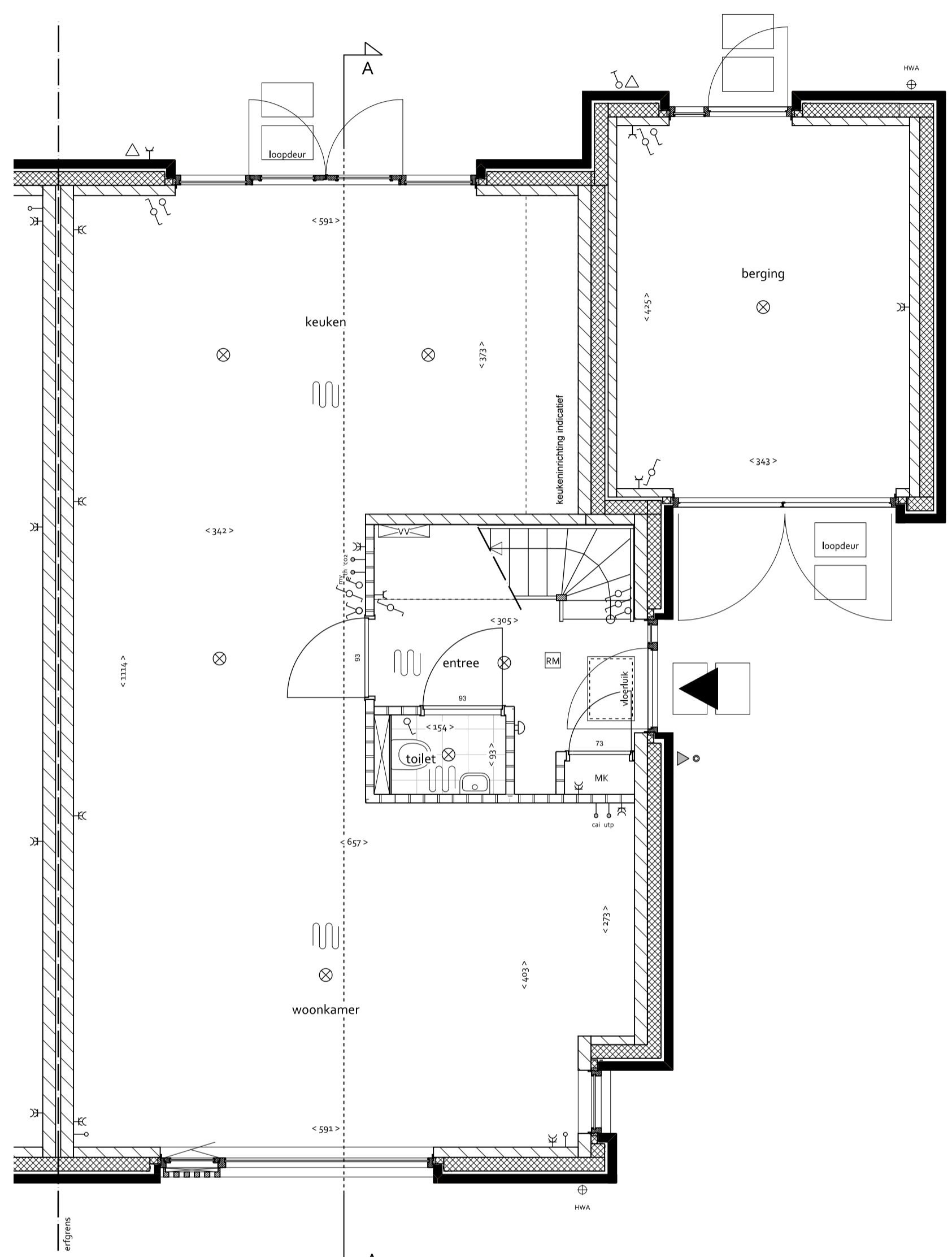
BEGANE GROND 1:50
