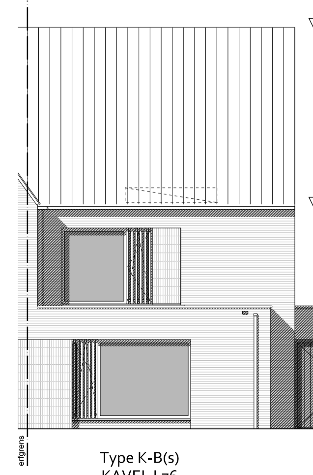
Type K-B(s) KAVEL L76 VOORGEVEL 1:100
