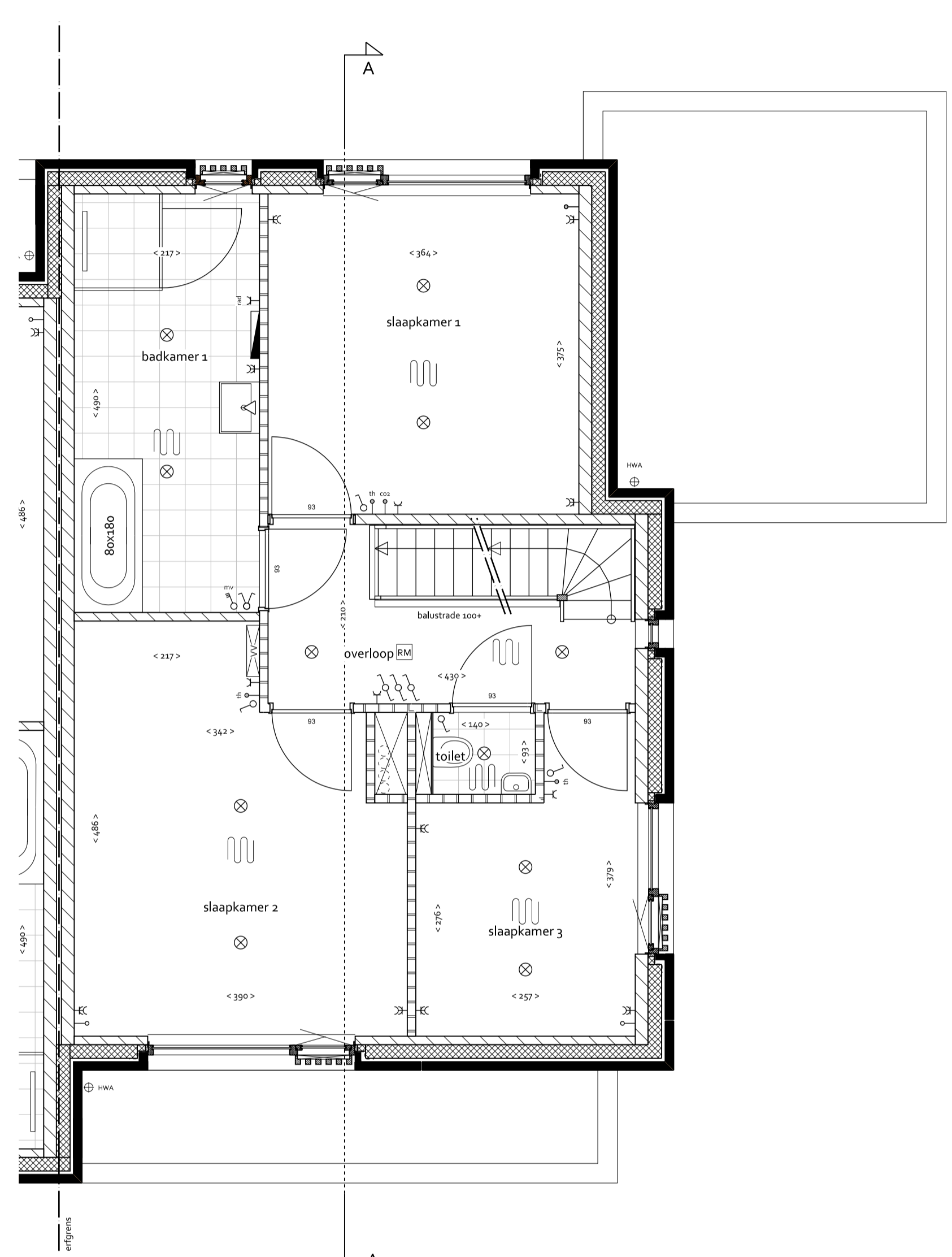
EERSTE VERDIEPING 1:50
