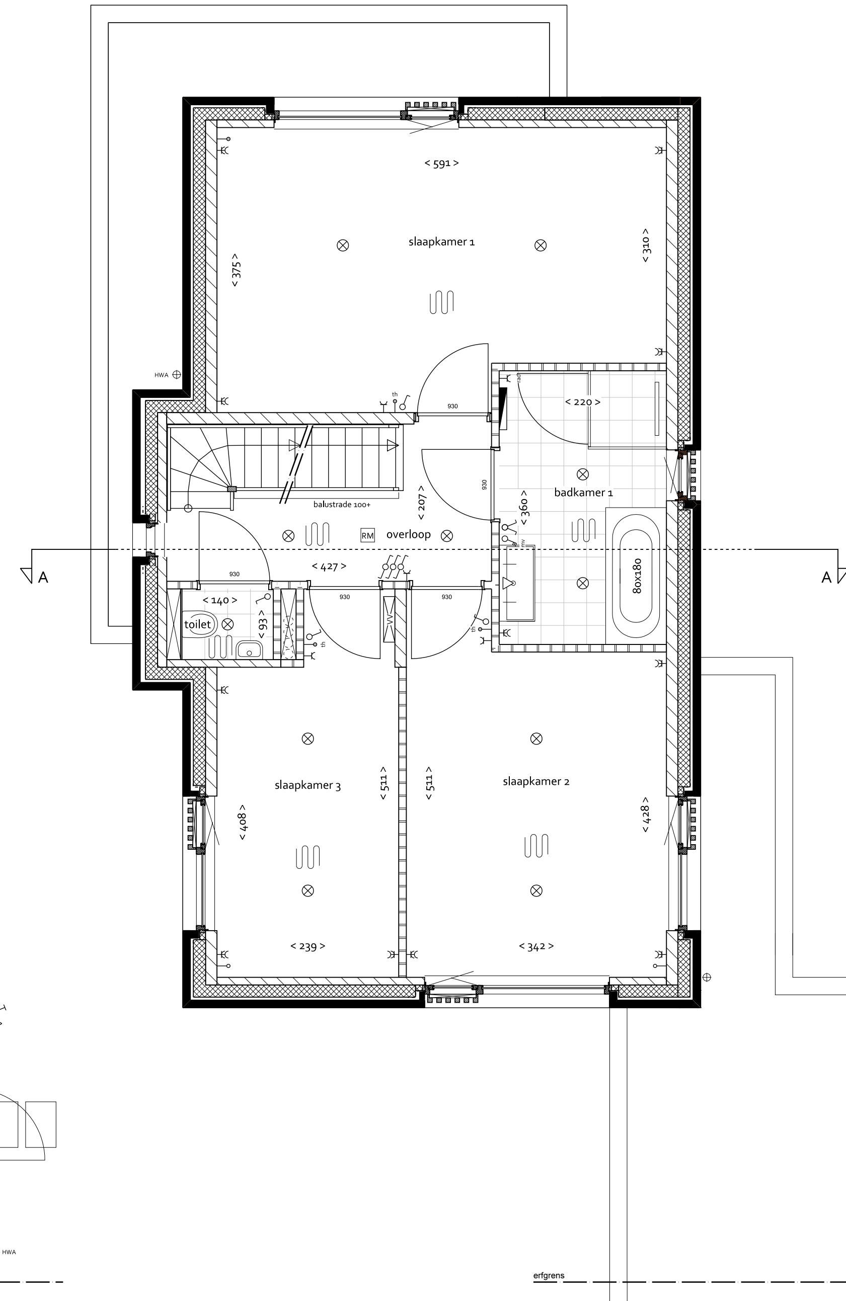
EERSTE VERDIEPING 1:50
