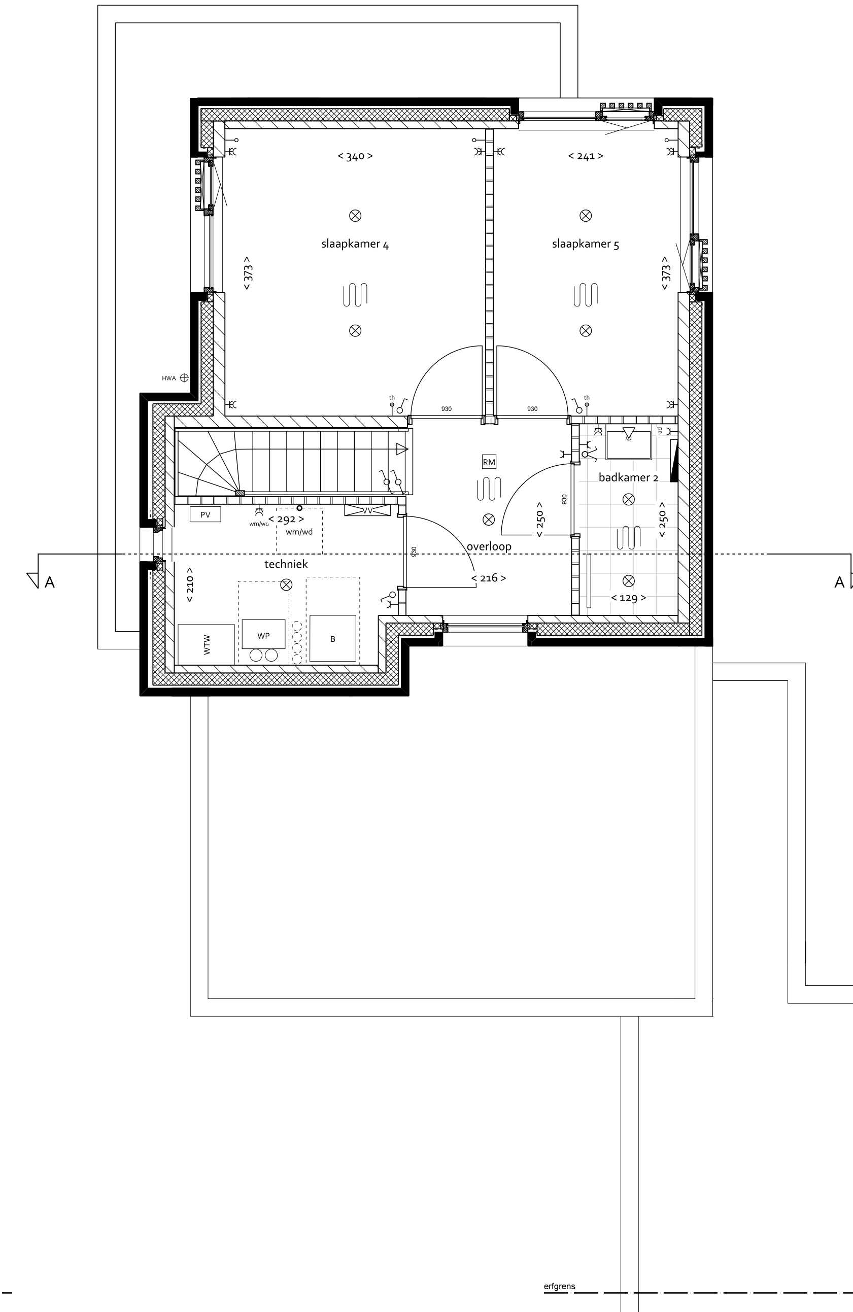
TWEDE VERDIEPING 1:50
