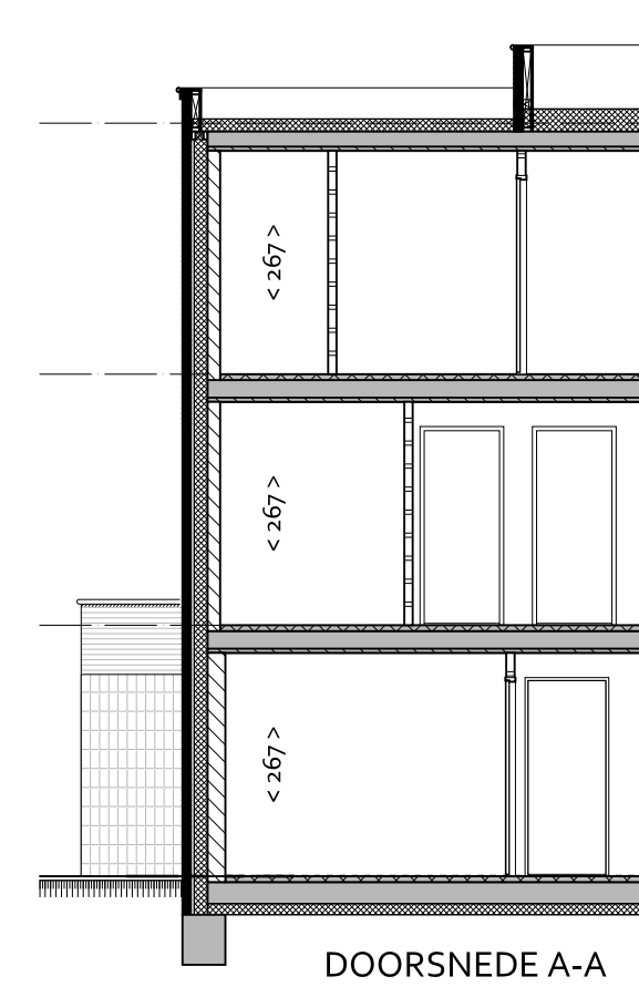
DOORSNEDE A-A 1:100
