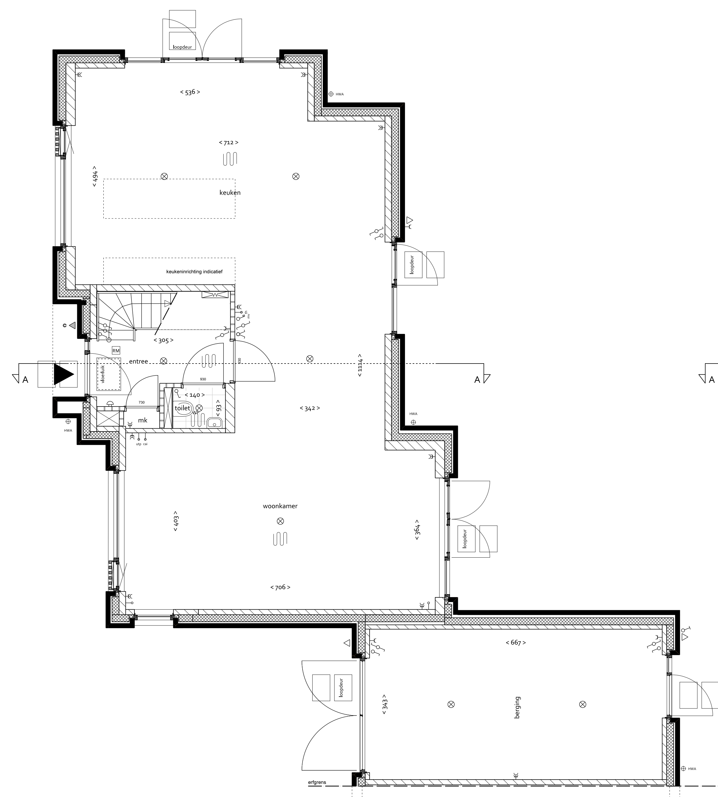
BEGANE GROND 1:50
