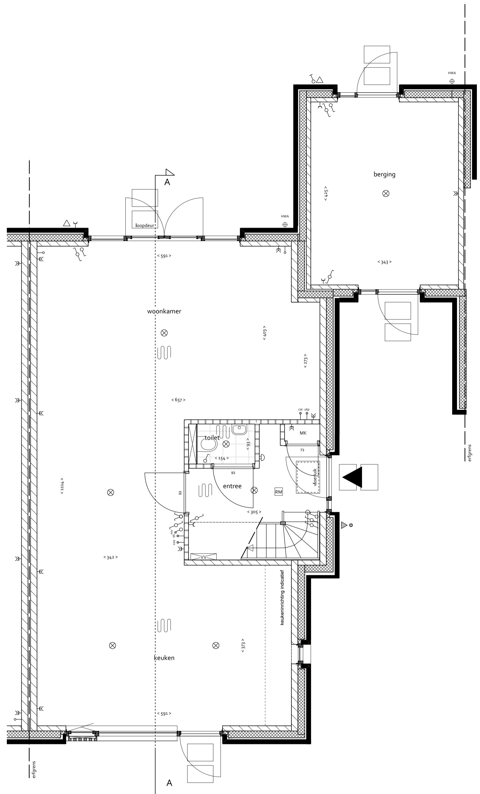
BEGANE GROND 1:50
