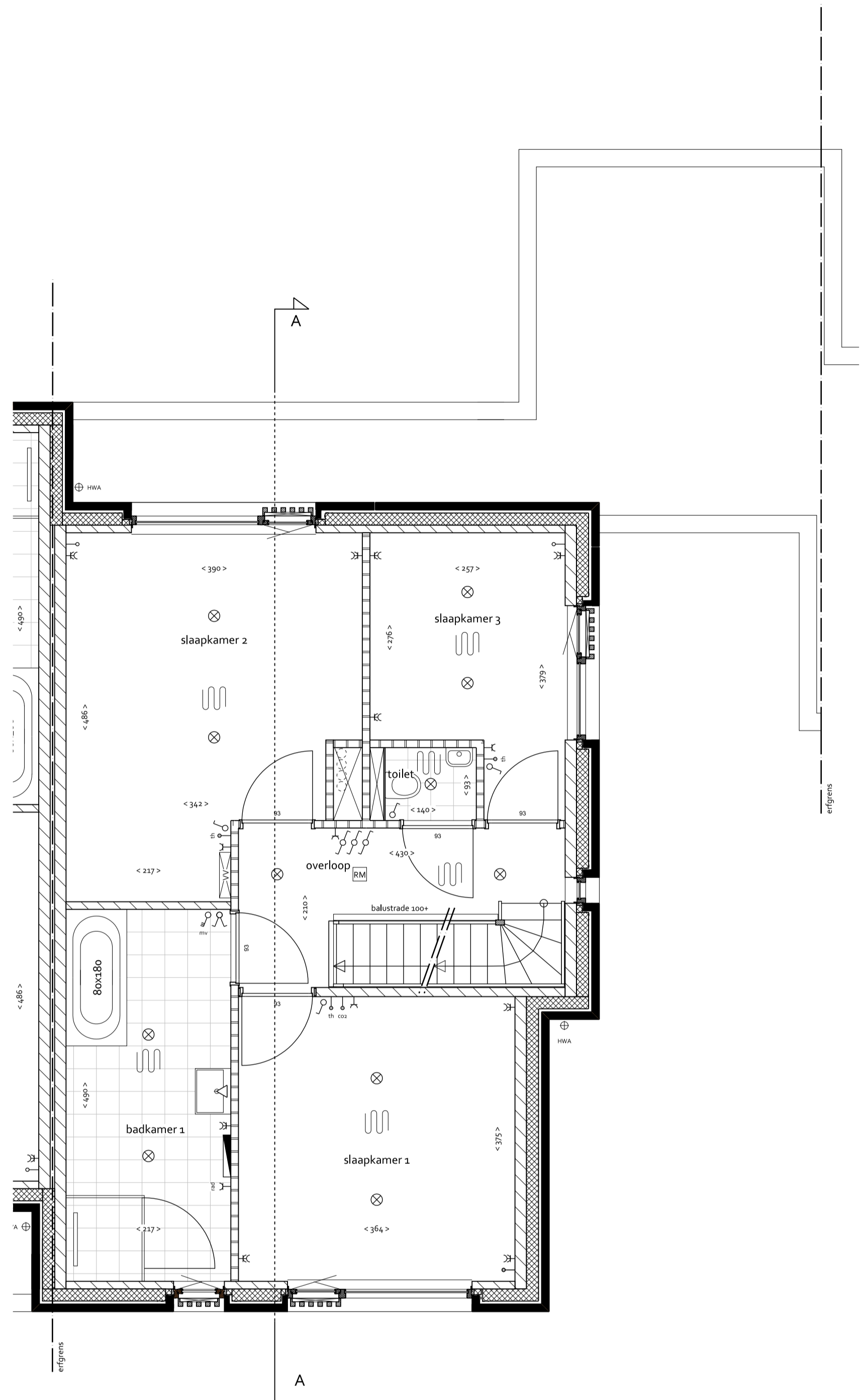
EERSTE VERDIEPING 1:50
