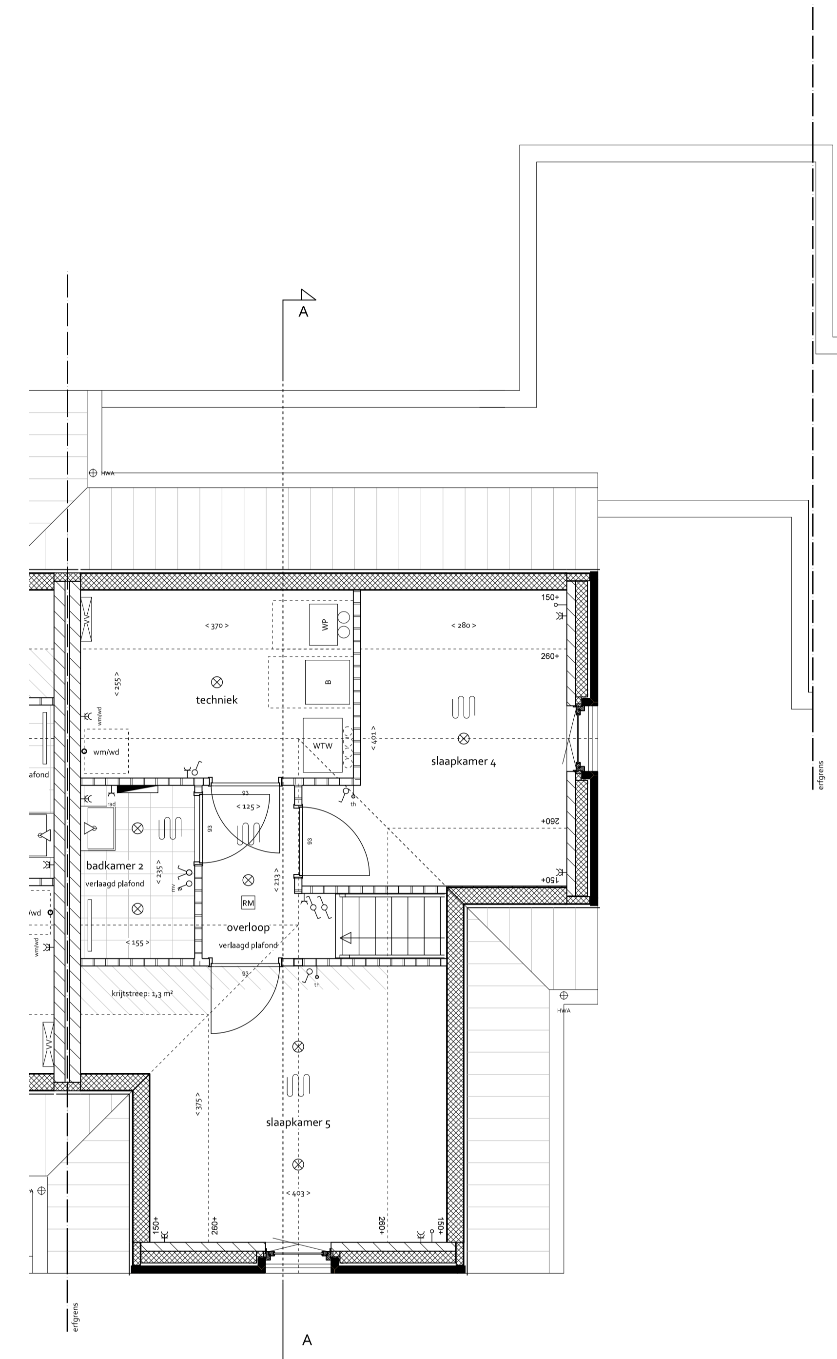
TWEEDE VERDIEPING 1:50
